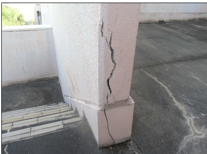
外部階段
